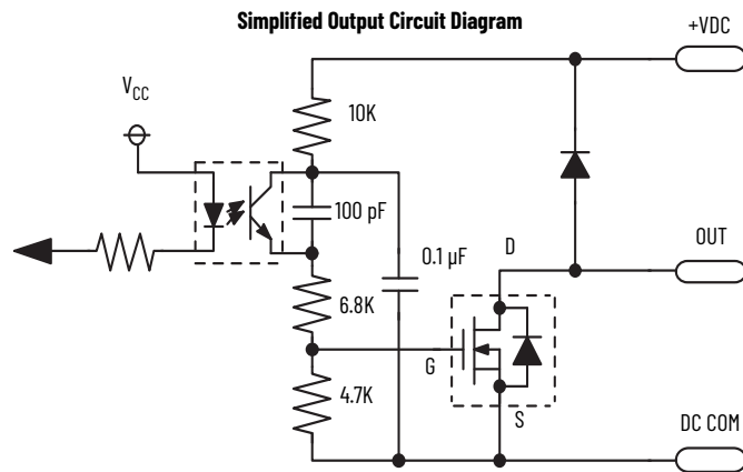
Output Wiring
