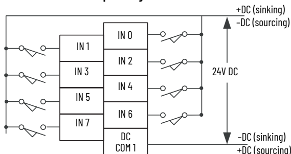
Input wiring
