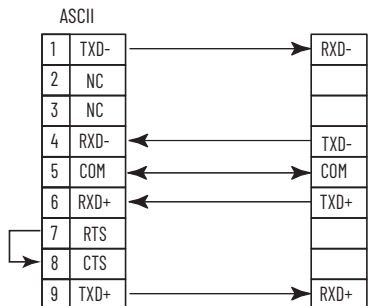
RS-422 Wiring
