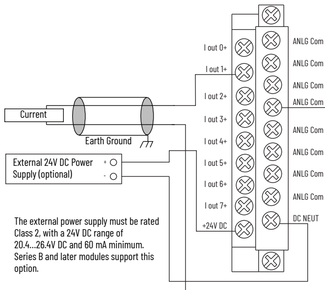
Output Wiring
