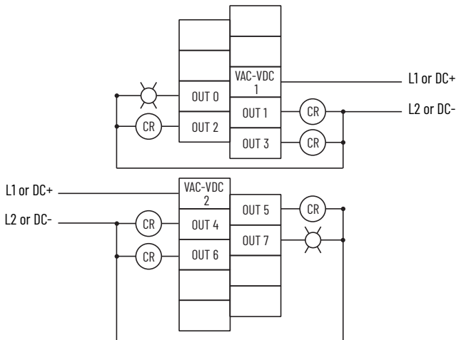
Output Wiring
