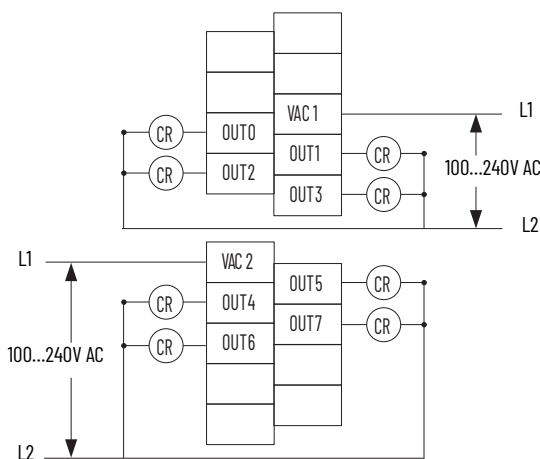
Output Wiring
