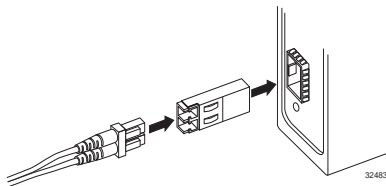
Fiber SFP Module
